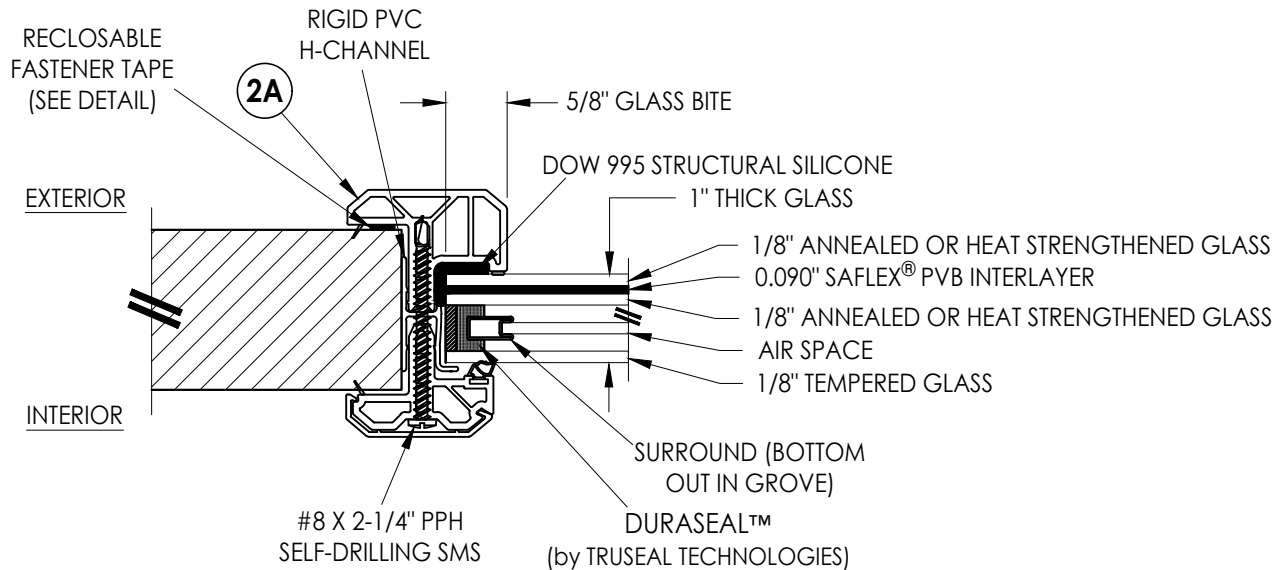
G2 GLAZING DETAIL DECOSEAL
